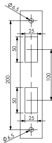
монтажен отвор
