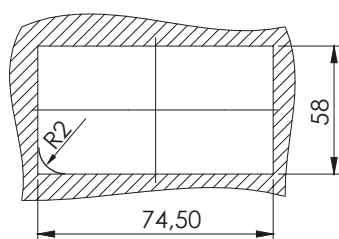
Монтажен отвор
