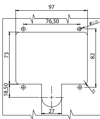
Монтажен отвор
