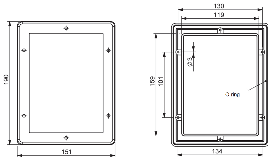
Версия 1 Закрепване чрез винтове
