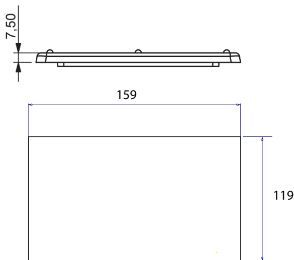
Монтажен отвор
