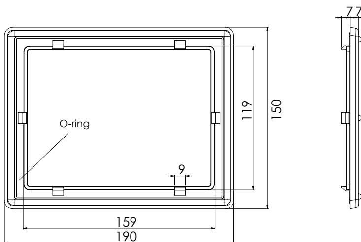
Версия 2 с клипсове не се изисква винт за закрепване
