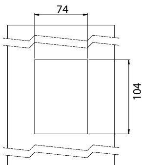
Посадочное отверстие
