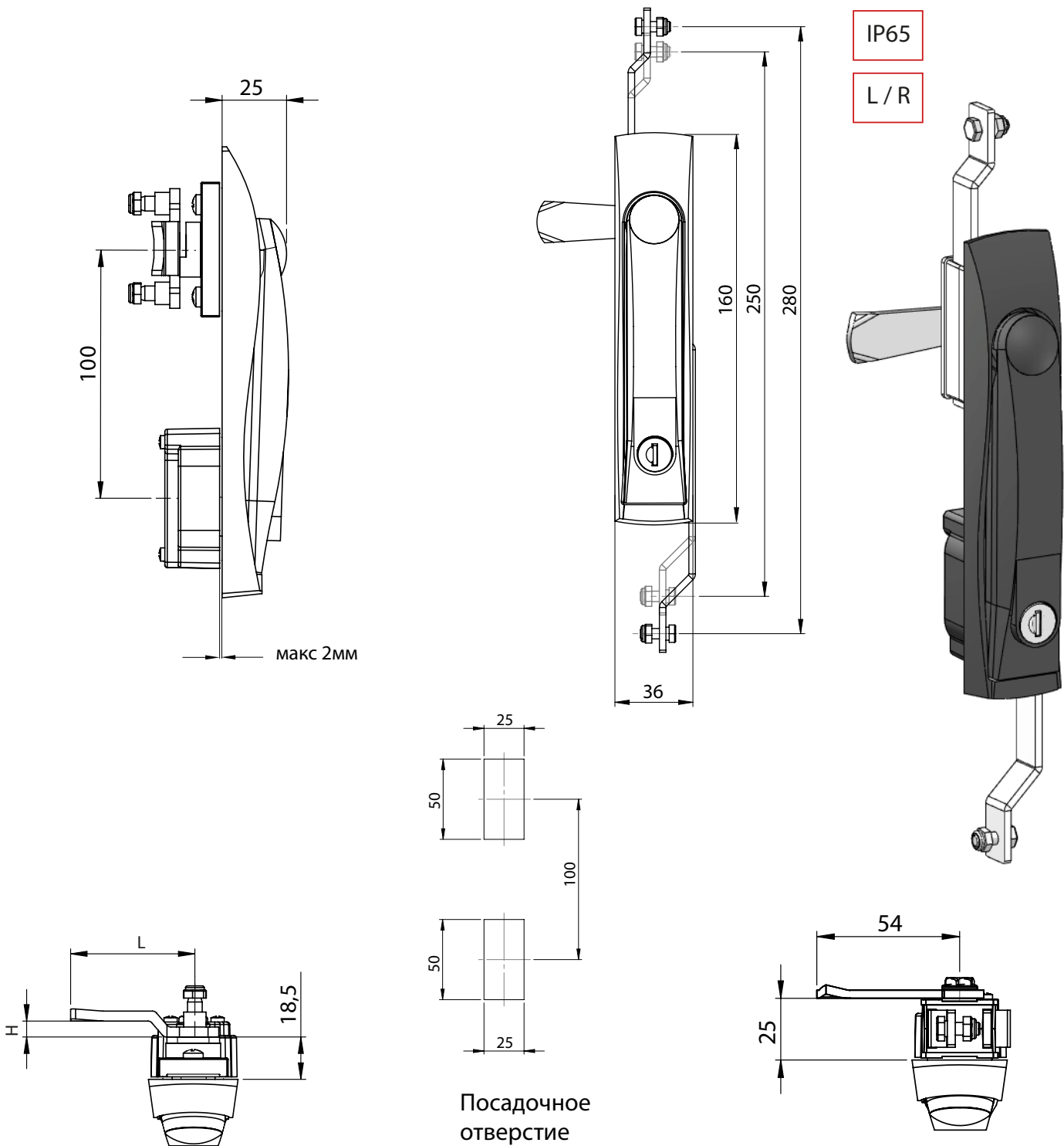
Вариант для языков с 3-точечным запираением - КК
