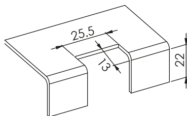
Монтажен отвор
