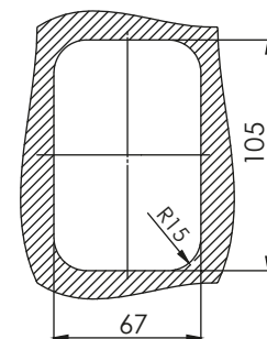
Монтажен отвор
