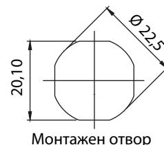
Монтажен отвор
