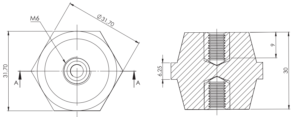
Подпорен изолатор SM (M6)
